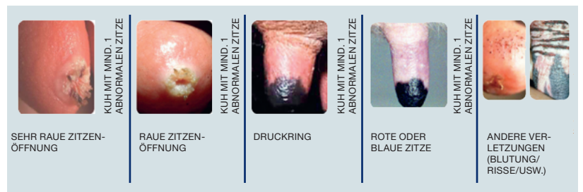
Abbildung 3: Zitzenbeurteilungskarte
